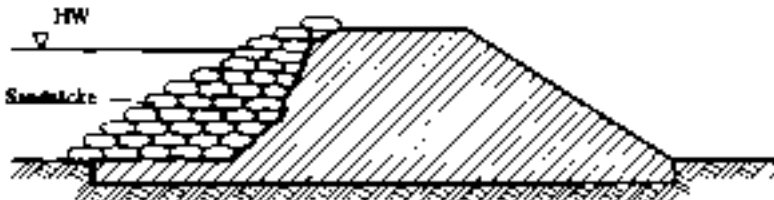
Abb. 22: Schadensstellenabdeckung mit Schüttsteinen und/oder Sandsäcken
