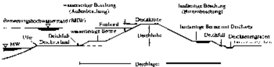
Abb. 11: Querschnitt eines Flussdeiches
