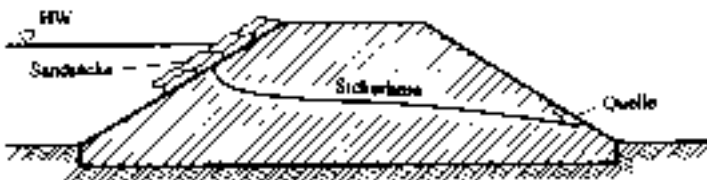
Abb. 28: Abdeckung einer Quelleneintrittsstelle
