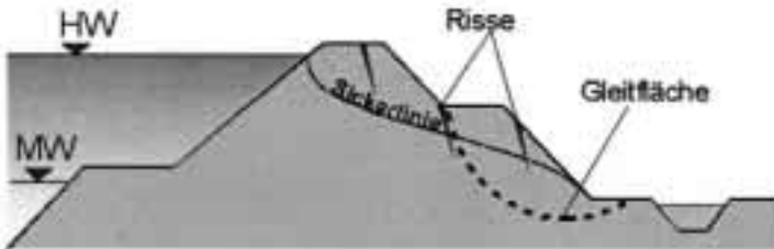
Abb. 31: Risse/beginnender Böschungsbruch
