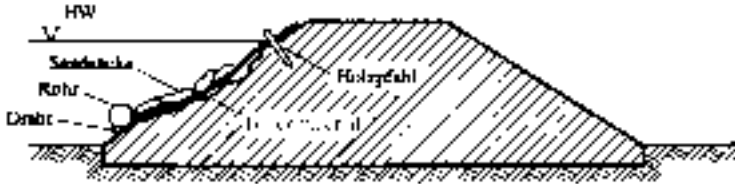
Abb. 21: Schadensstellenabdeckung durch Aufbringen von Folienmaterial
