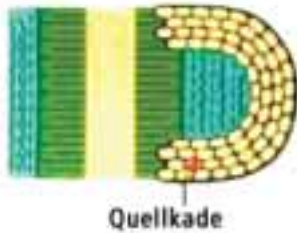
Abb. 29: Fangedamm
